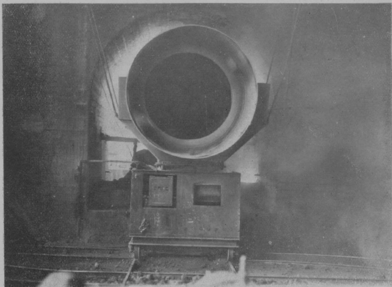
小野田セメント工場 (その五) セメント焼塊の冷却筒を出る状況
