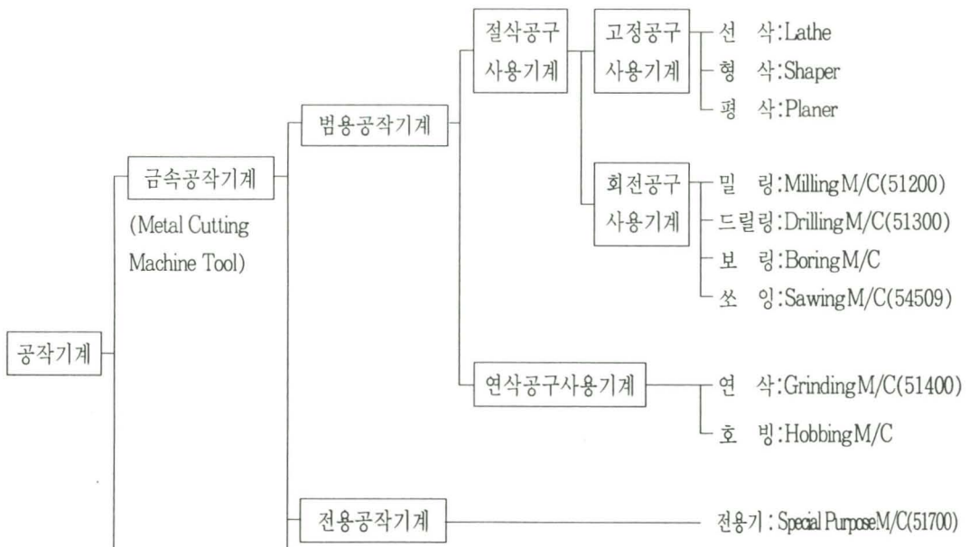
공작기계의 분류
