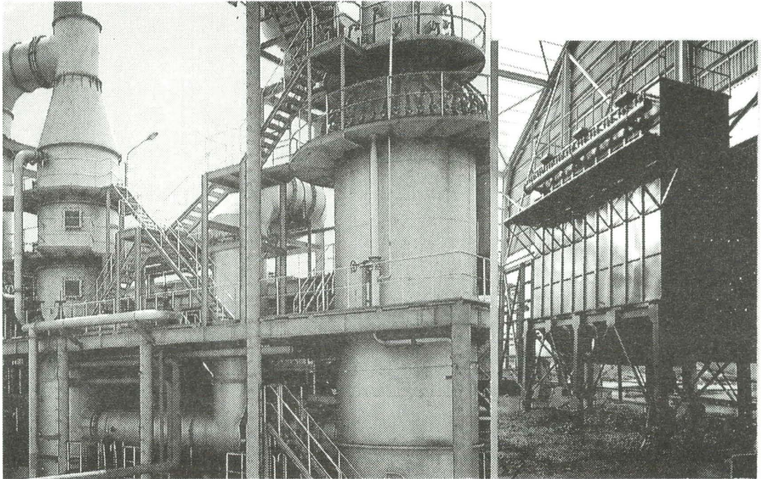
집진장치
