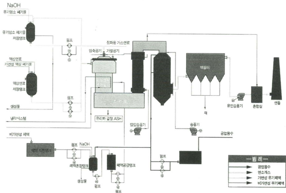
소각설비 공정흐름도
