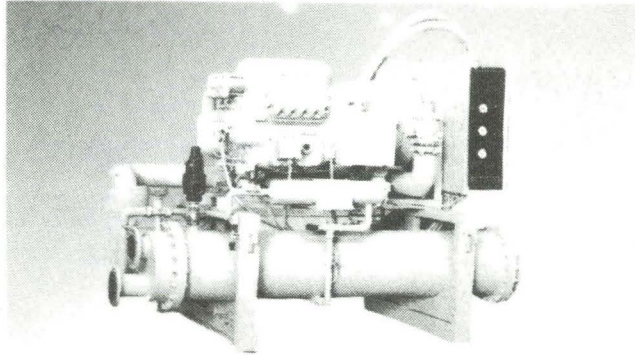
왕복식 냉동기
