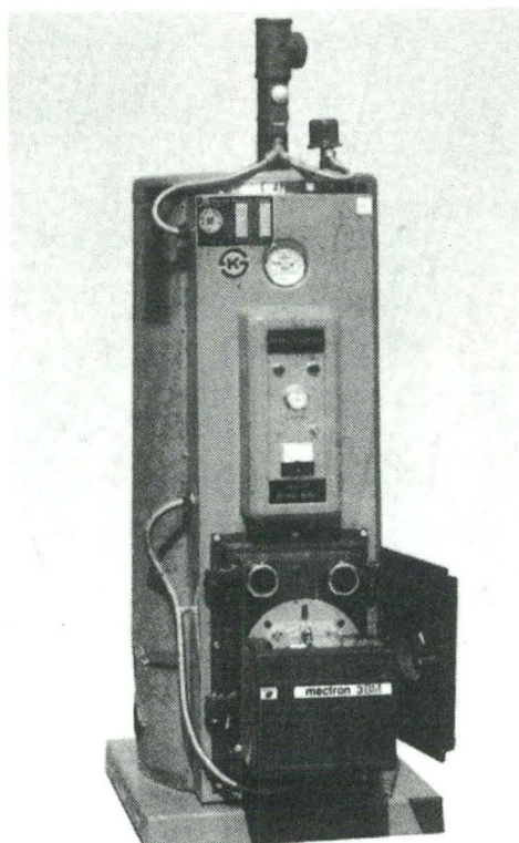
온수 보일러
