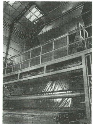
〈필름 생산설비〉
