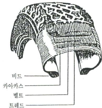
래디알타이어 구조
