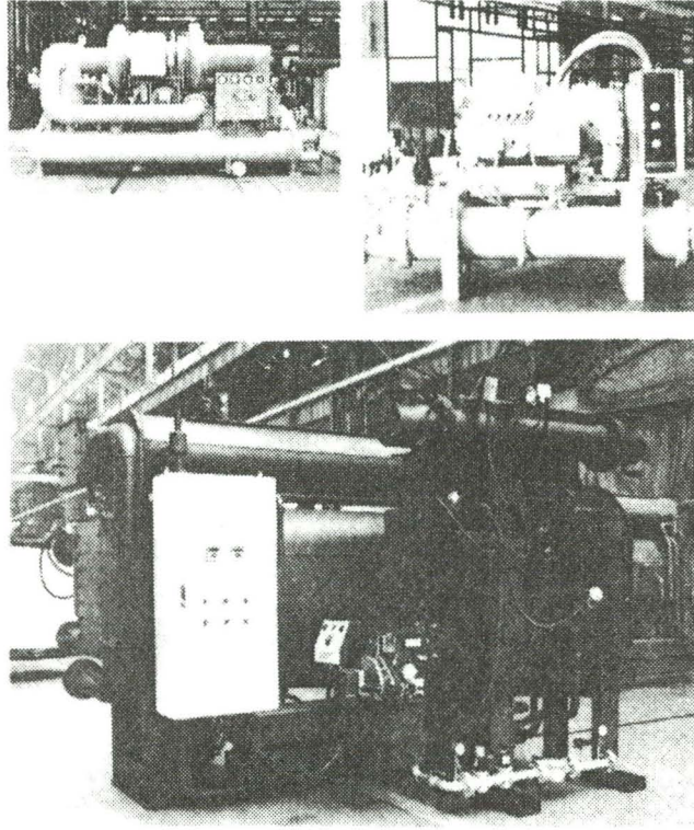
냉매용 공기압축기
