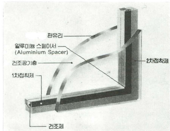
복층유리단면도
