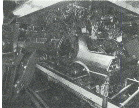
용접용 로봇
